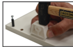
D. Con un martillo colocar la escuadra de fijación
