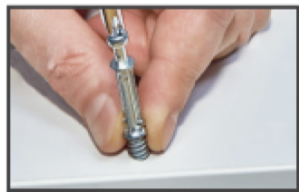
D. Atornillar pernos minifix
