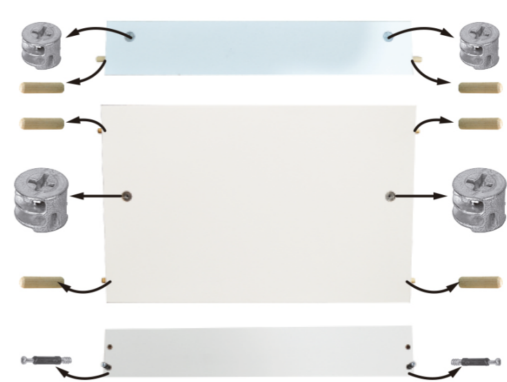
A. Encolar en todas las uniones entre piezas
