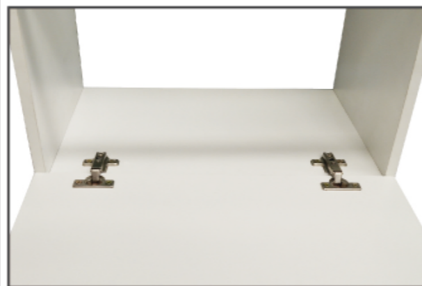
A. Regule la posición de las puertas ajustando los tornillos de regulación de las bisagras.
